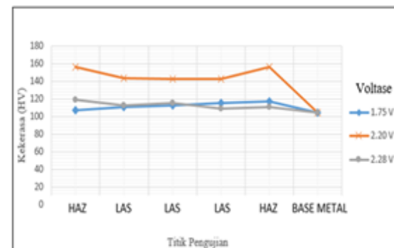
Gambar 9 Grafik pengujian kekerasan 3 lapis
