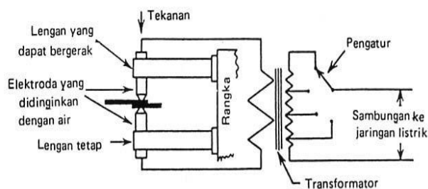
Gambar 3 Diagram Alat Las Titik
