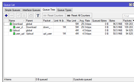
Gambar 5.. Traffic upلود dan download pada Queue Tree
