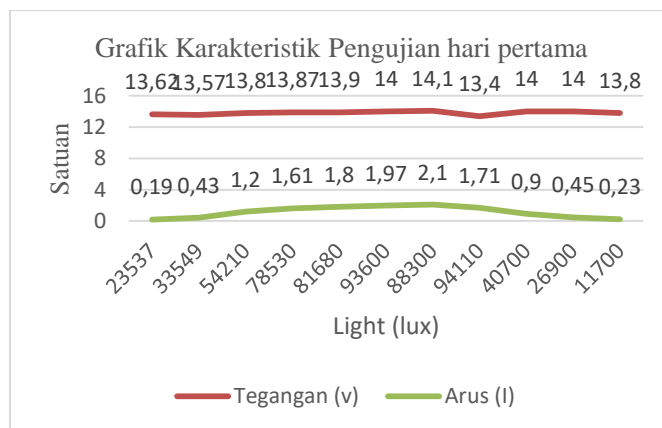
Grafik 3 Pengaruh Intensitas Cahaya Terhadap Tegangan dan Arus pada output solar charger pada pengukuran
