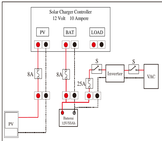
Gambar 2 Diagram Instalasi Pengawatan KAPASITAS PANEL SURYA
