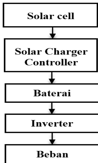
Gambar 1 Diagram Blok Sistem Kerja PLTS
