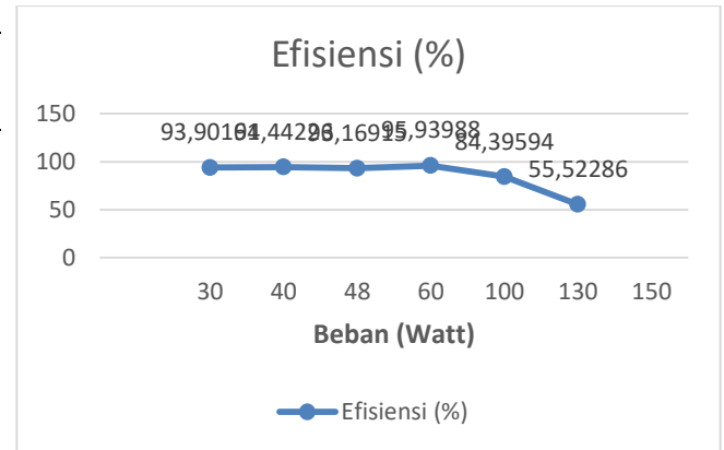
Grafik 5 Grafik efisiensi inverter untuk beban
