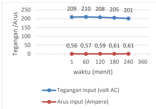
Grafik 7 Grafik hubungan tegangan dan arus output inverter dengan beban
