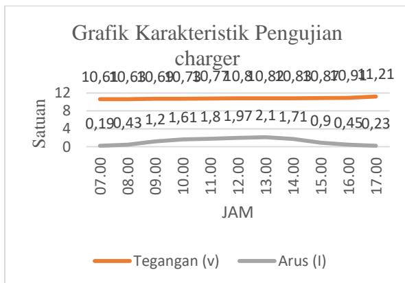
Grafik 4. Tegangan Dan Arus Charger
