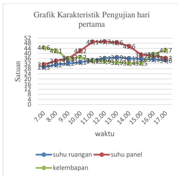
Grafik 1 Pengaruh suhu dan kelembapan terhadap waktu pada pengukuran
