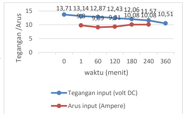
Grafik 6 Grafik hubungan tegangan dan arus input inverter dengan beban
