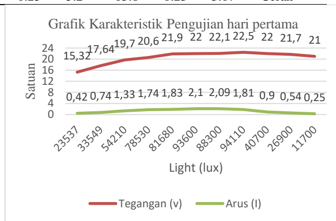
Grafik 2 Pengaruh Intensitas Cahaya Terhadap Tegangan dan Arus pada Output Solar Cell pada pengukuran
